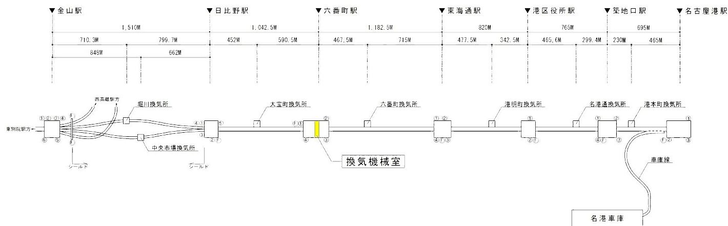
名港線路線図 ①～⑥：駅出入口 F：換気口
