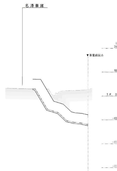
車庫線縦断面図 縦横比 40 : 1
